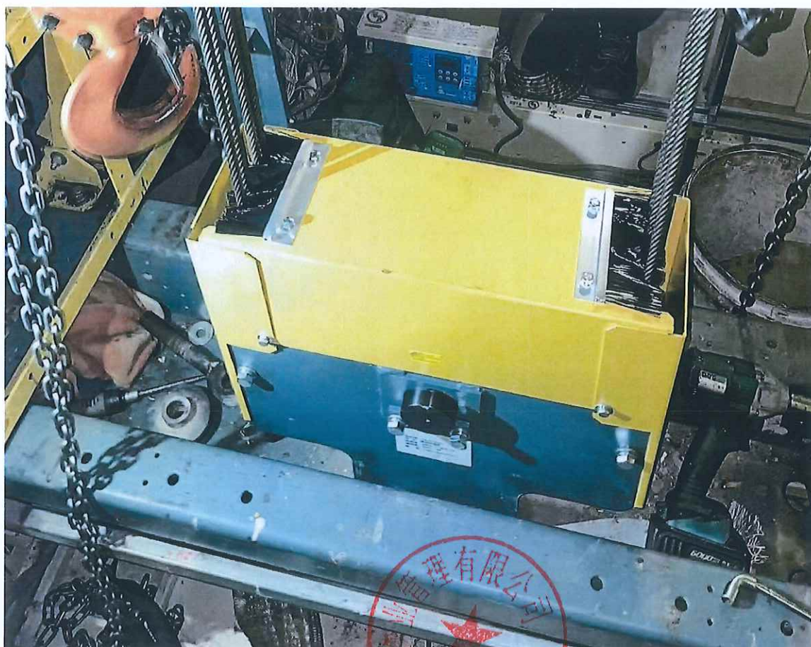
轿顶反绳轮更换后
