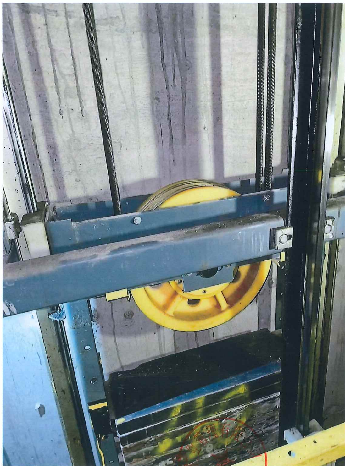
对重反绳轮更换前
