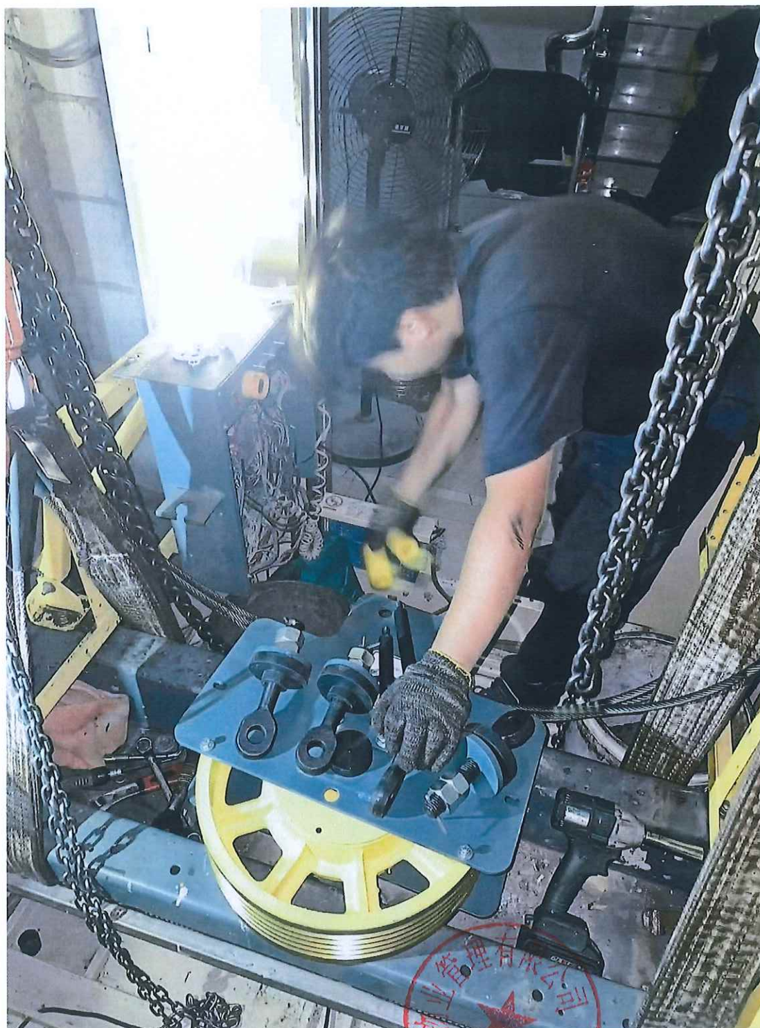
对重反绳轮更换中
