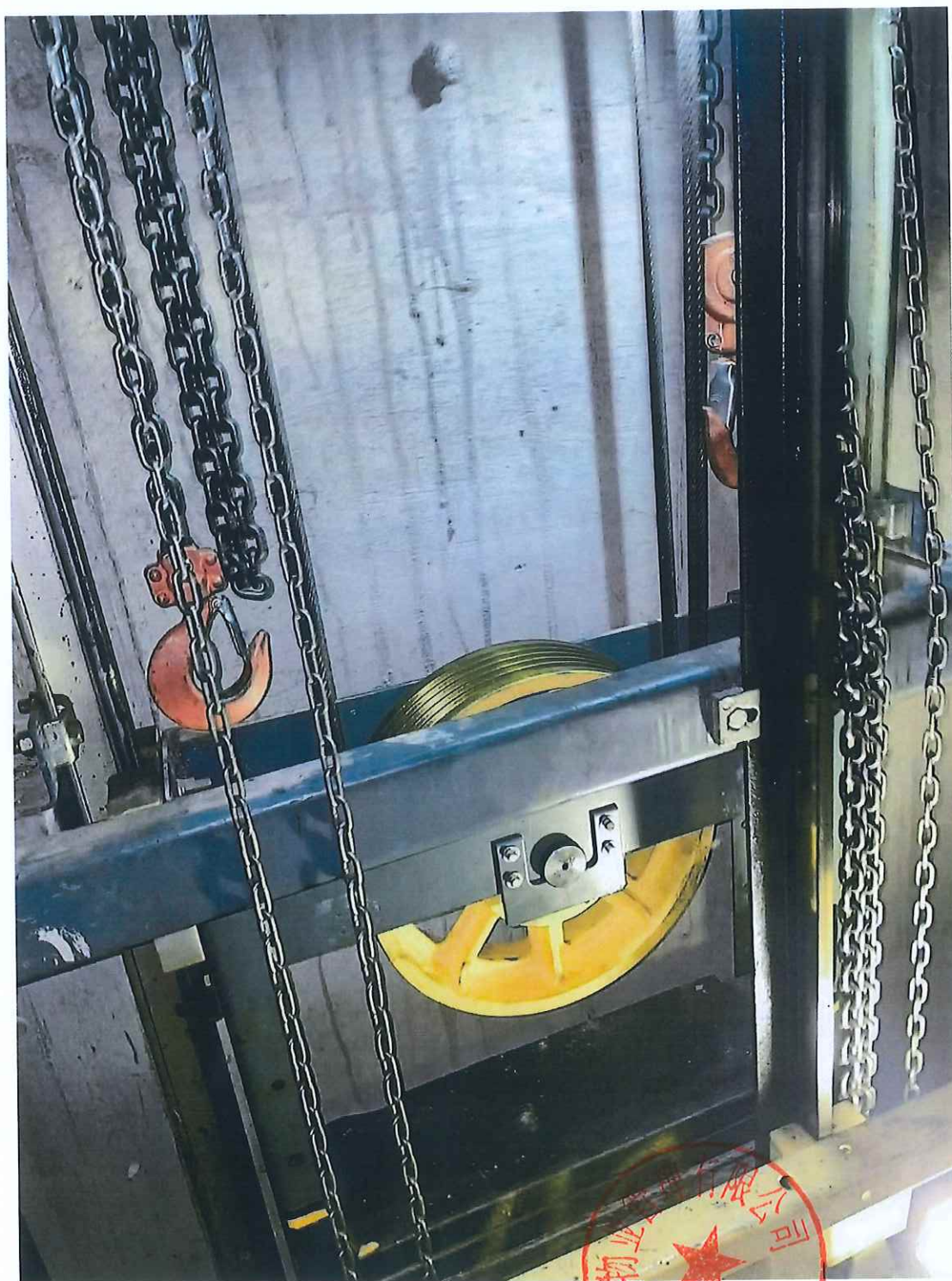
对重反绳轮更换后
