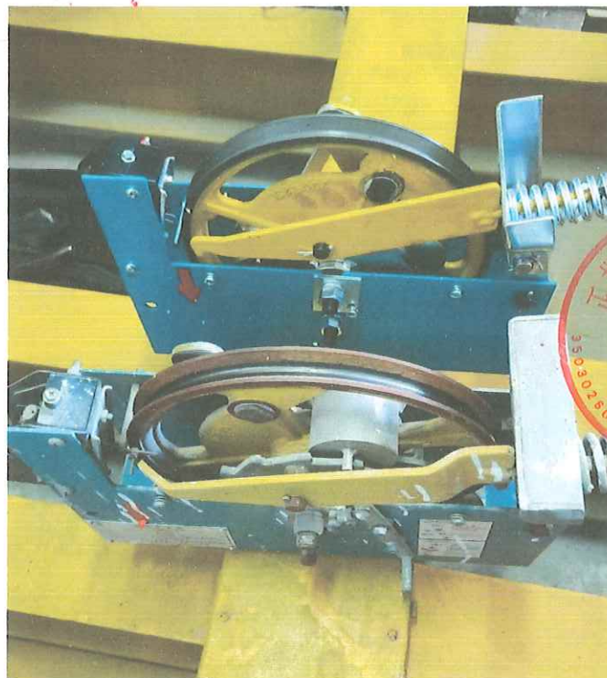
限速器更换中
