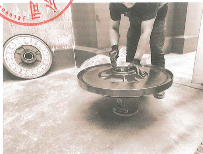
曳引轮更换中
