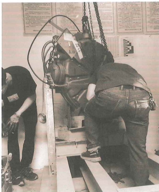
曳引轮更换中
