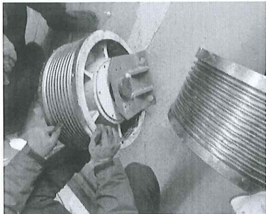
机房导向轮更换中
