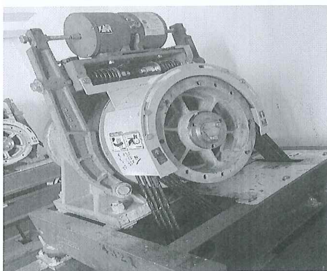
曳引机调心滚子轴承、深沟球轴承更换后
