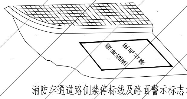
消防车通道沿线禁停标线及路面警示标志示例
